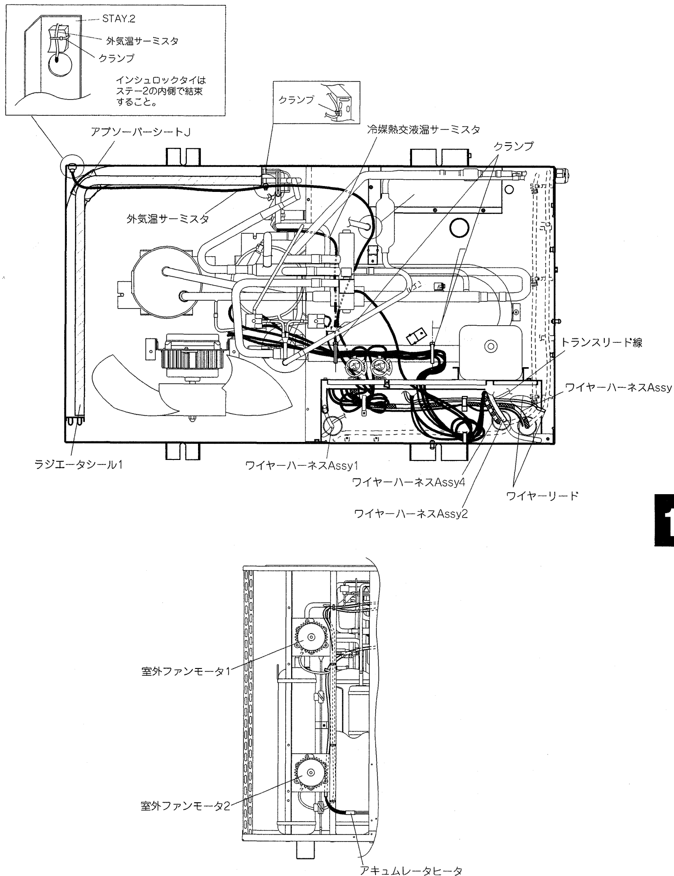
(熱交ルーム内ハーネス取回し図)
