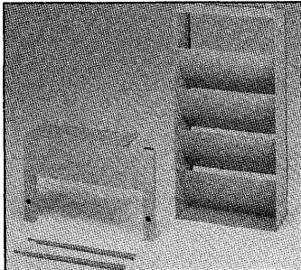
風向変更板 室外ユニットファンからの風の吹出方向を変える事ができます。室外ユニットが道路や隣家に面している場合やベランダ設置などに効果を発揮します。 注) 風向変更板取付けにより5%程度能力低下する場合があります。
