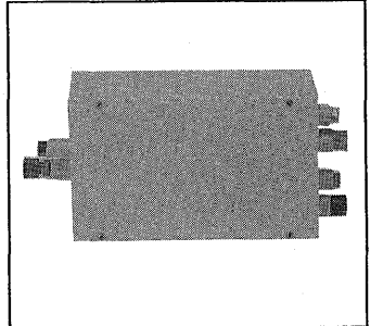
分岐ユニット 室外ユニット冷媒1系統を2つに分岐することができます。 室外ユニット1台あたり分岐ユニット3台まで接続可能です。
