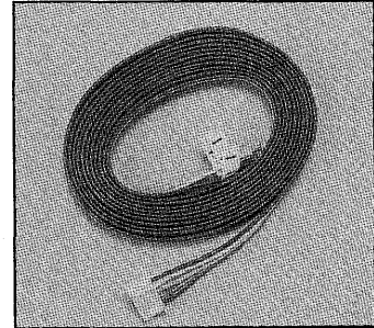
遠方表示用アダプタ 監視盤等から出力されるパルス信号により、エアコンの一括ON/OFF操作と監視盤への運転/異常の表示取出しができます。
