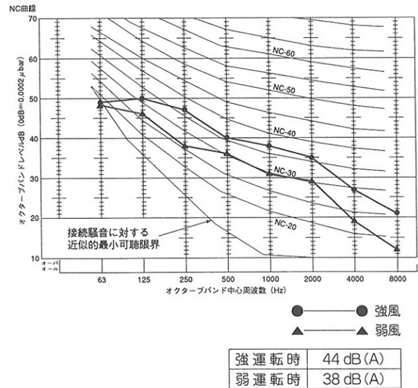
●YMEJ140B-A1 (標準円形ダクト仕様35Pa下吸込仕様)
