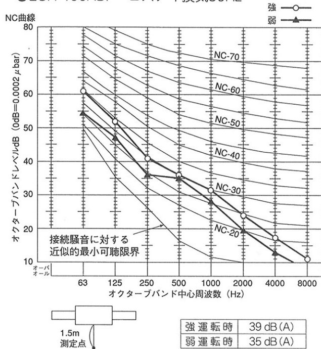
● LGH-100RDF ロスナイ換気50Hz
