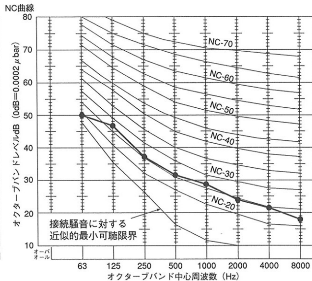
●YMEJ112・J140D-B1-F(オールフレッシュ仕様130Pa)
