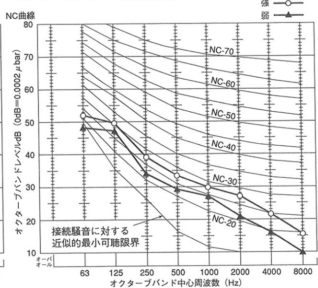
●LGH-80RDF 普通換気60Hz
