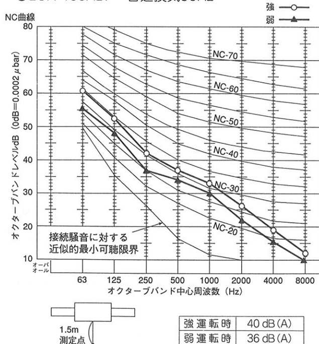
● LGH-100RDF 普通換気50Hz
