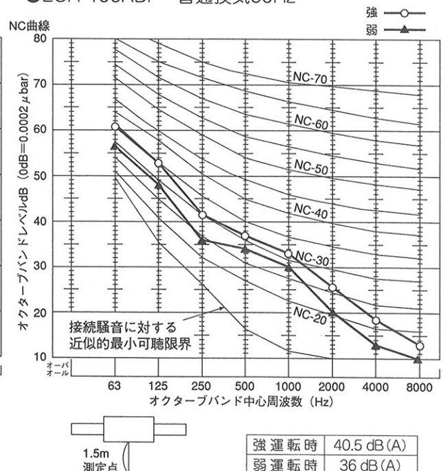
● LGH-100RDF 普通換気60Hz
