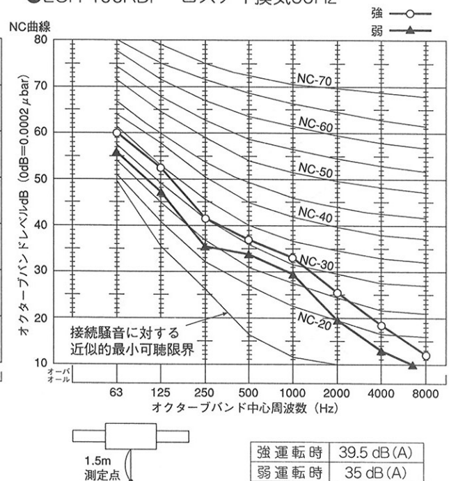
● LGH-100RDF ロスナイ換気60Hz
