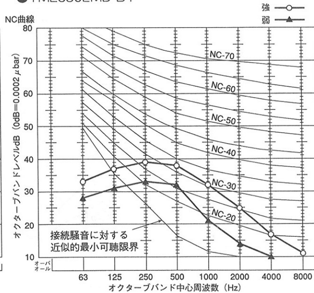
●YMEJ80LMD-B1
