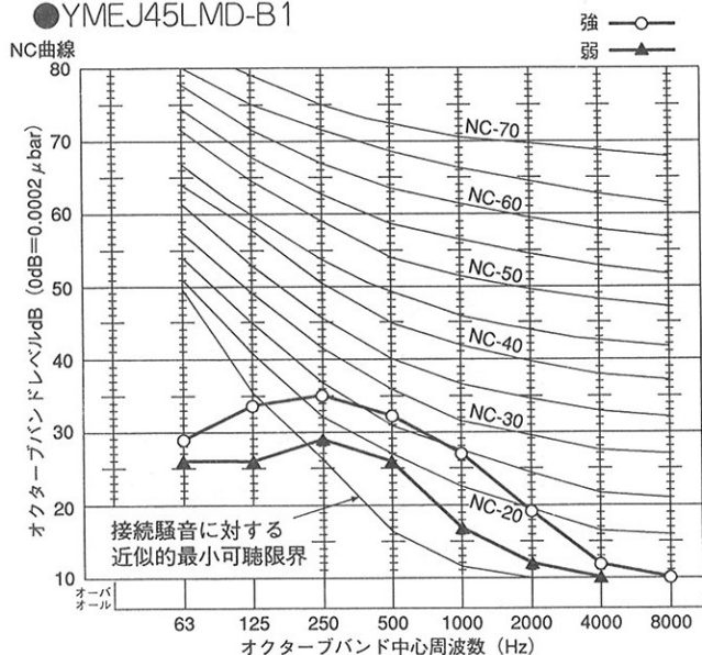
●YMEJ45LMD-B1
