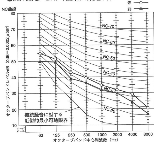
●LGH-80RDF ロスナイ換気(SA吹き出し斜め45° 1.5m)50Hz
