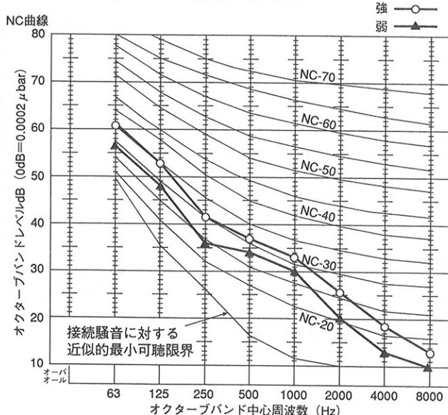
●LGH-100RDF 普通換気60Hz
