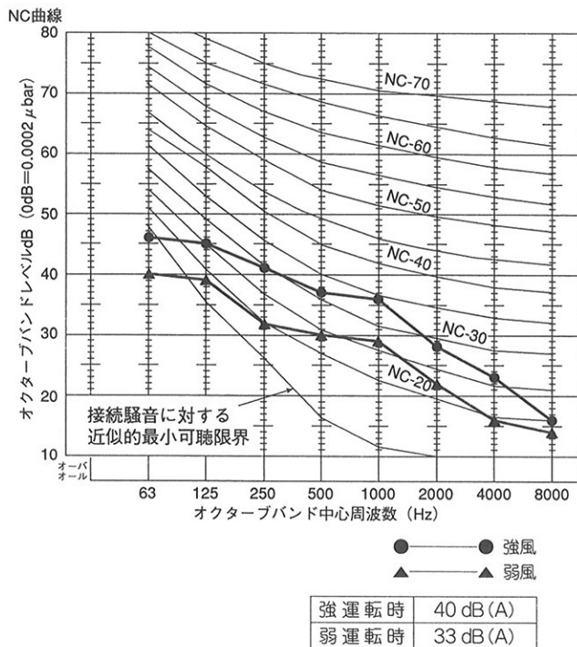
●YMEJ71D-B1(100Pa)
