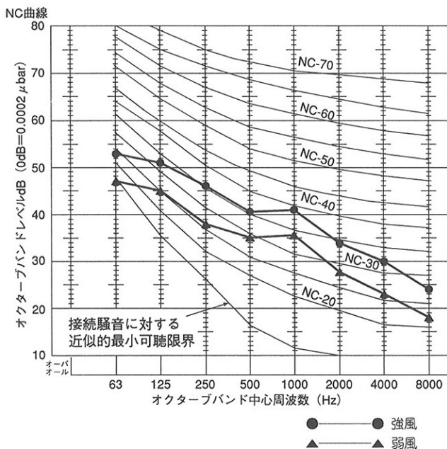
●YMEJ71D-B1(200Pa)
