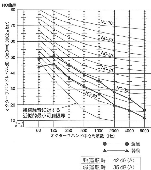
●YMEJ90D-B1(100Pa)
