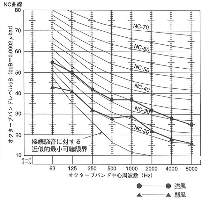
●YMEJ56D-B1(200Pa)
