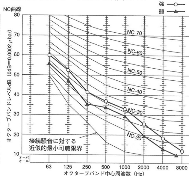
●LGH-100RDF ロスナイ換気60Hz
