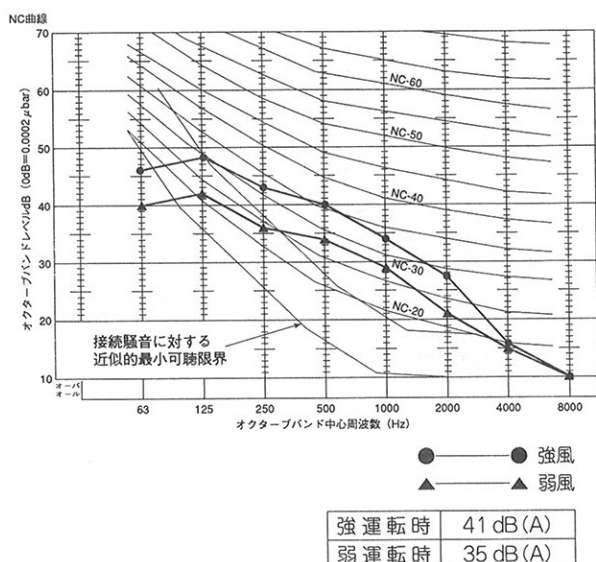
●YMEJ80B-A1 (標準円形ダクト仕様35Pa下吸込仕様)
