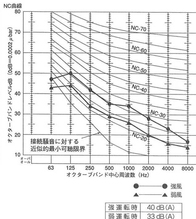
●YMEJ80D-B1(100Pa)
