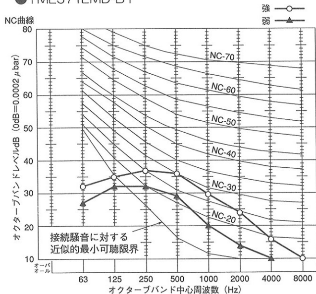
●YMEJ71LMD-B1
