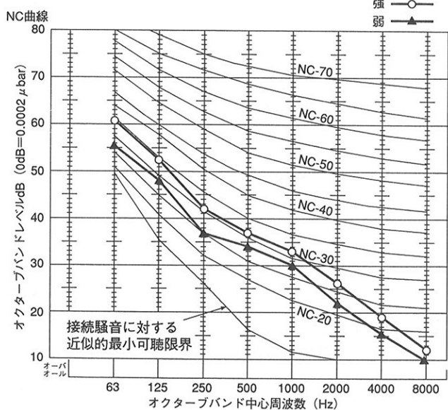
●LGH-100RDF 普通換気50Hz
