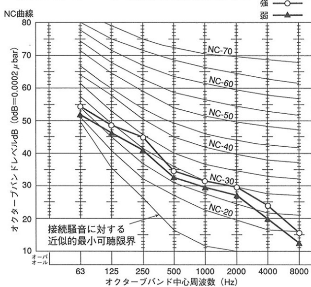
●LGH-50RDF ロスナイ換気(SA吹き出し斜め45° 1.5m) 50Hz
