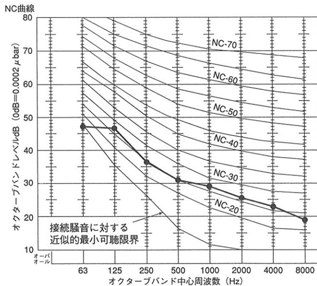
●YMEJ90D-B1-F(オールフレッシュ仕様130Pa)
