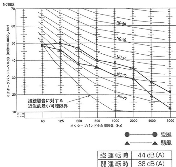
●YMEJ140B-A1 (標準円形ダクト仕様35Pa下吸込仕様)
