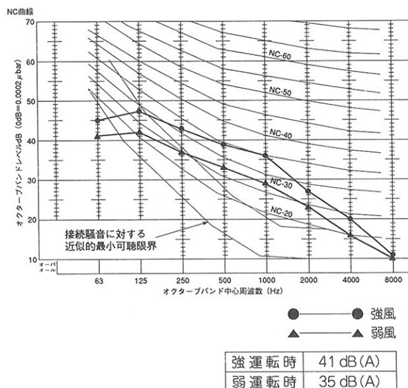
●YMEJ90B-A1 (標準円形ダクト仕様35Pa下吸込仕様)
