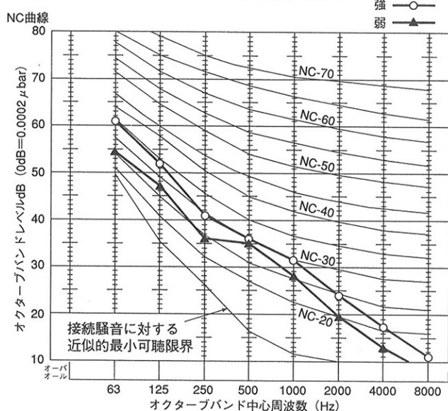
●LGH-100RDF ロスナイ換気50Hz
