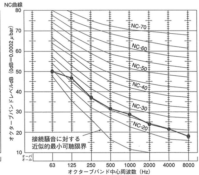
●YMEJ112・J140D-B1-F(オールフレッシュ仕様130Pa)
