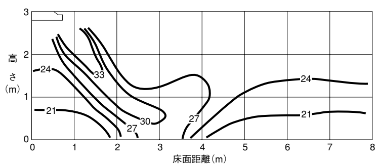
J71 暖房 下吹き出し 風量：強ノッチ 吹出角：60°
