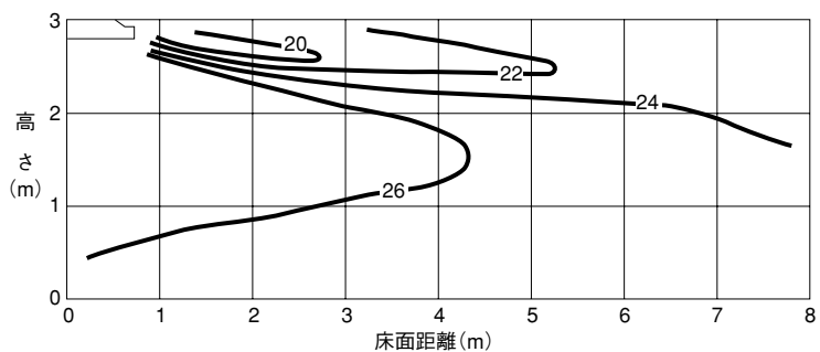
J140 冷房 水平吹き出し 風量：強ノッチ 吹出角：0°
