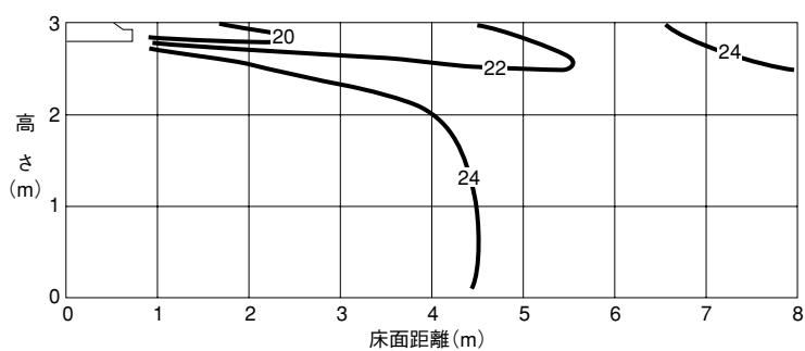
J71 冷房 水平吹き 風量：強ノッチ 吹出角：0°
