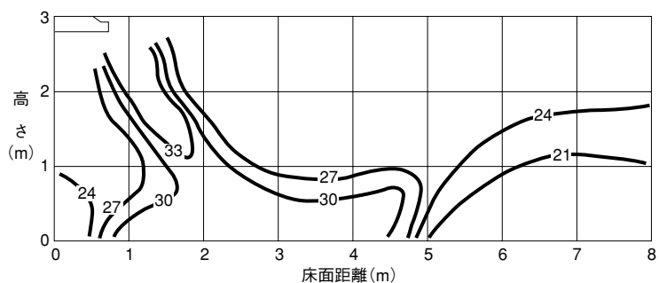
J140 暖房 下吹き出し 風量：強ノッチ 吹出角：60°
