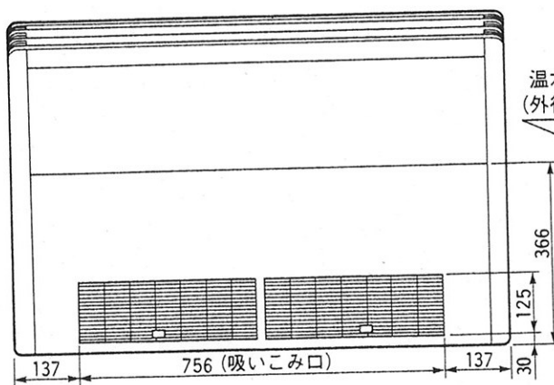
下面図
