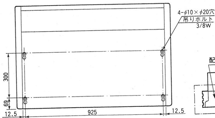
上面図
