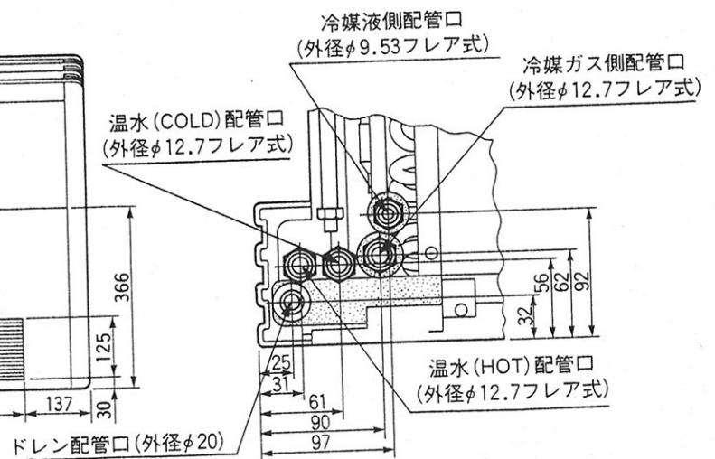
枠内詳細
