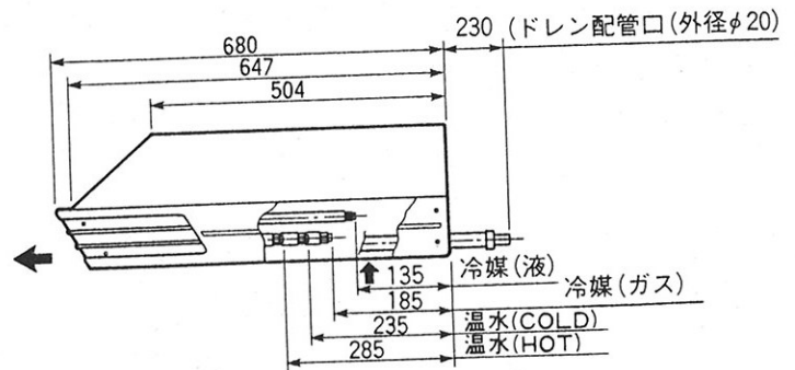
右側面図
