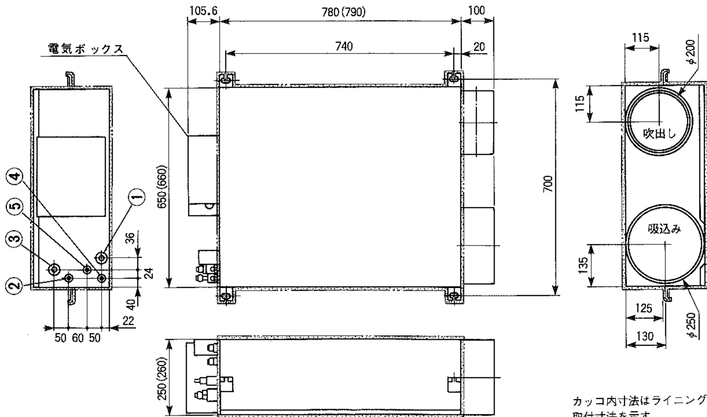
YGE401DW-2 (UT型)
