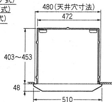
右側面図
