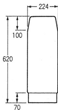
側面図
