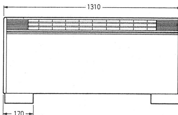
正面図
