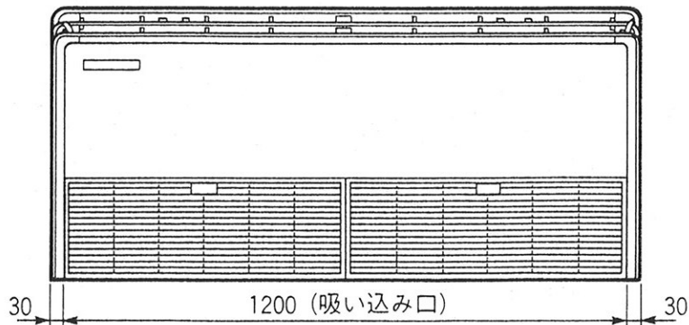
下面図
