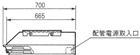
右側面図
