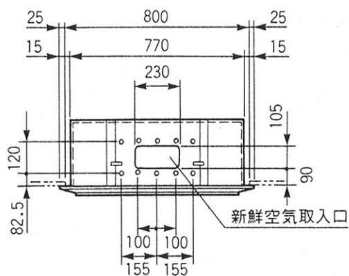
左側面図
