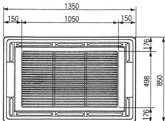
底面図
