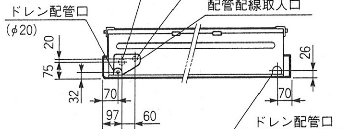
背面図
