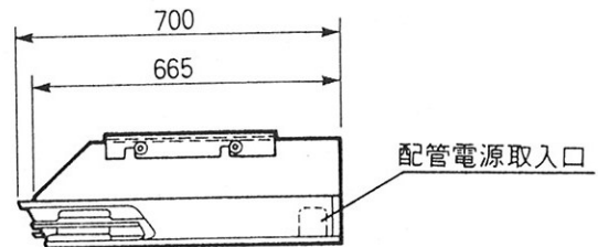
右側面図
