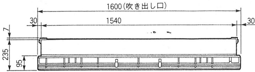
正面図
