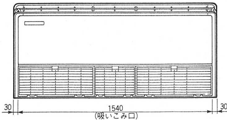
下面図
