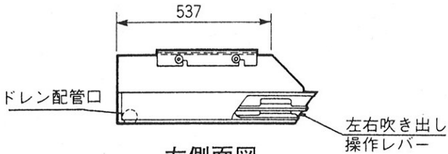
左側面図
