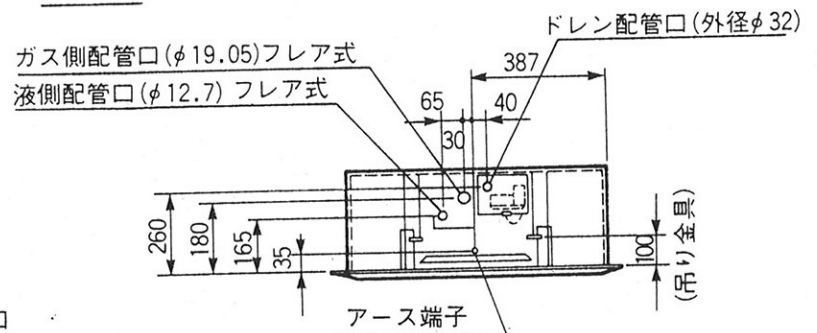
右側面図
