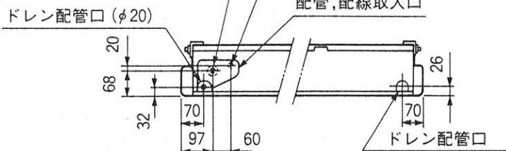
背面図
