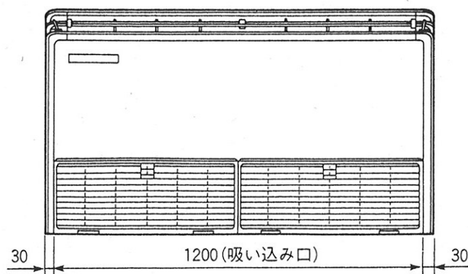
下面図
