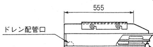
左側面図
