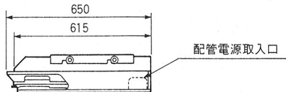
右側面図
