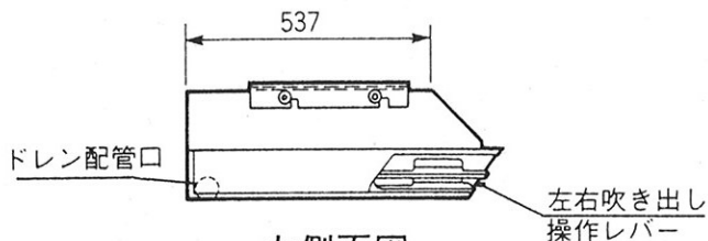
左側面図
