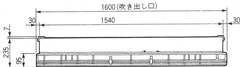
正面図
