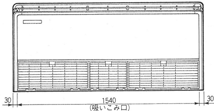
下面図
