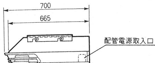
右側面図
