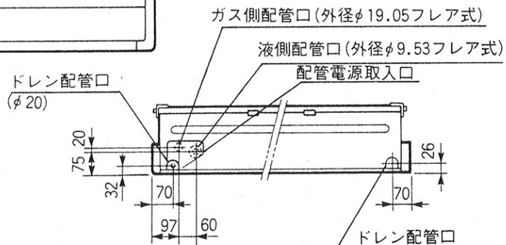
背面図
