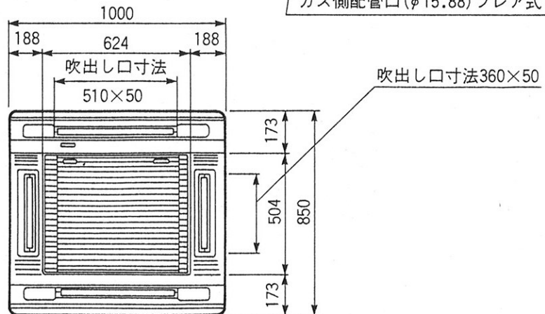
底面図
