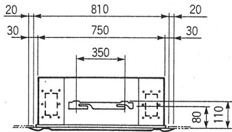
左側面図
