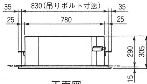
正面図
