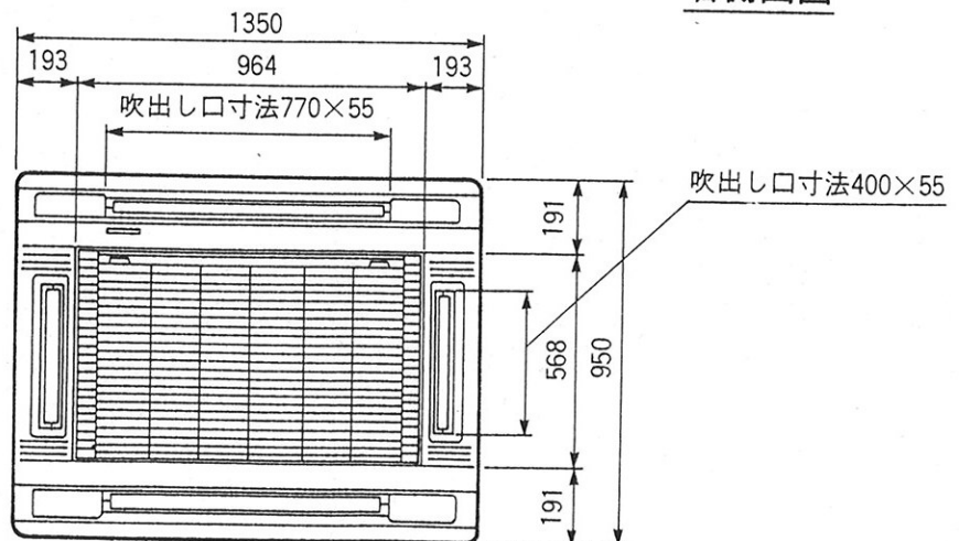
底面図
