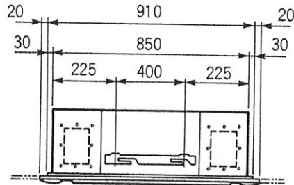
左側面図
