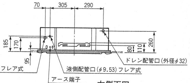
右側面図
