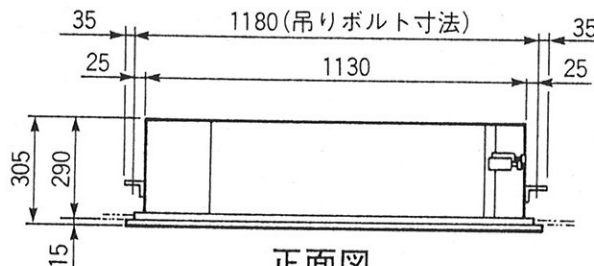
正面図
