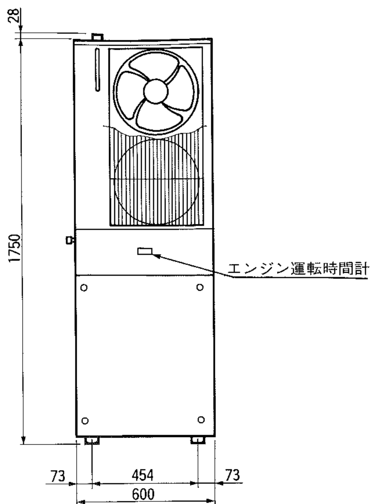
正面図
