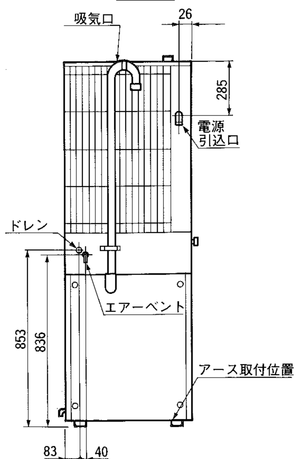
正面図
