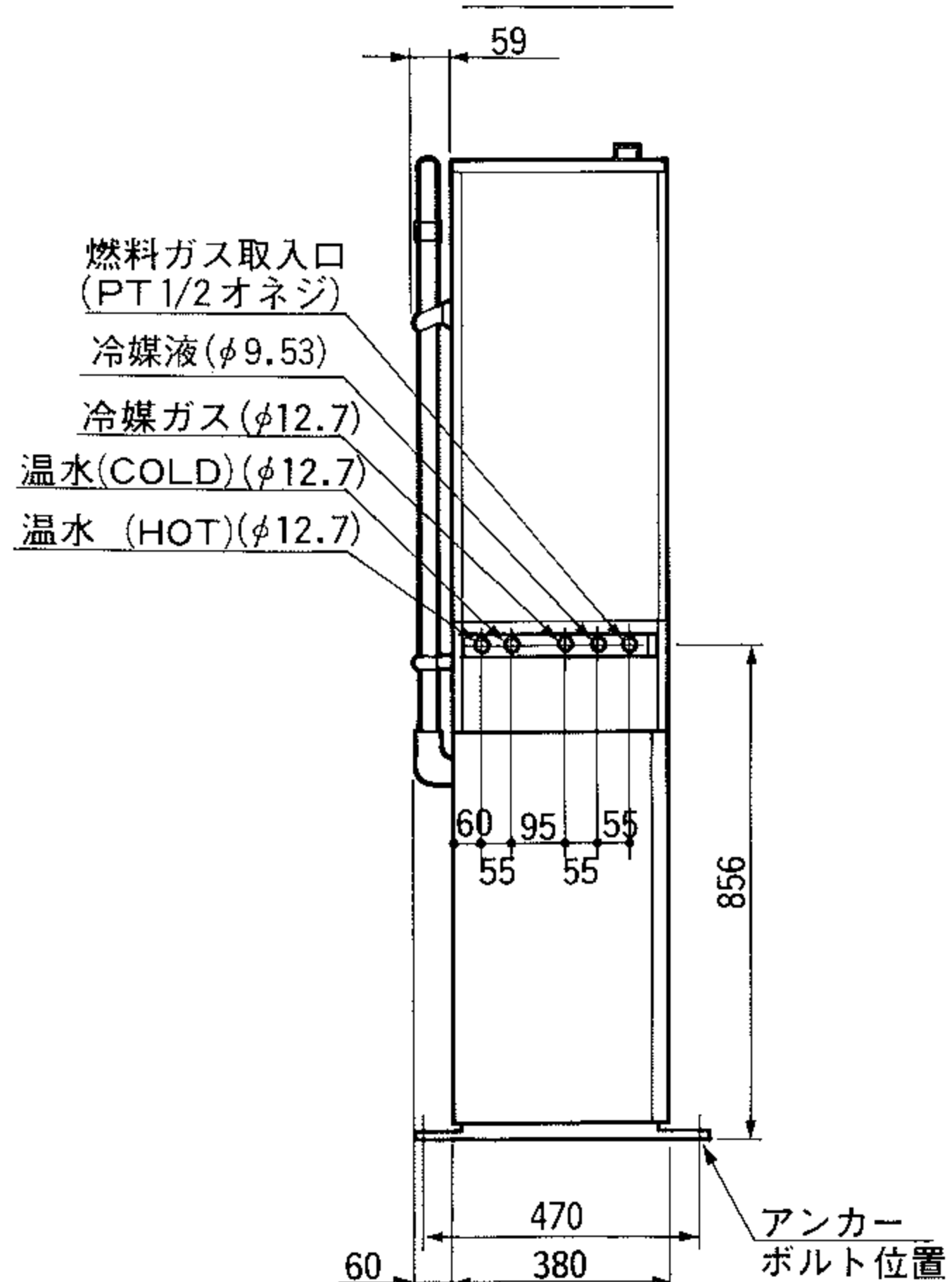
左側面図
