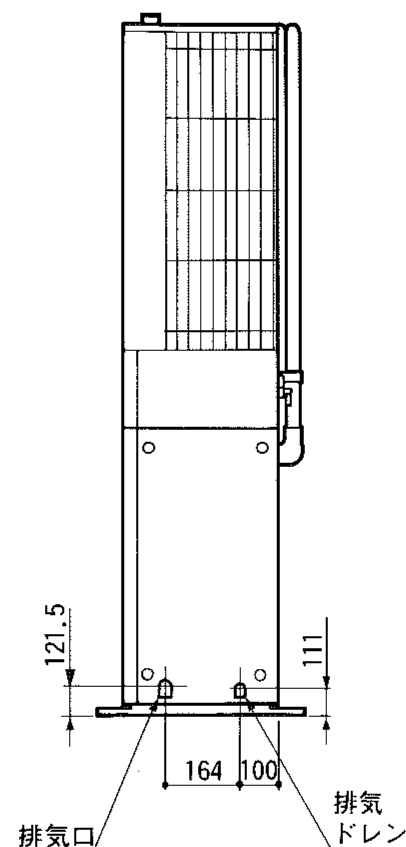
右側面図
