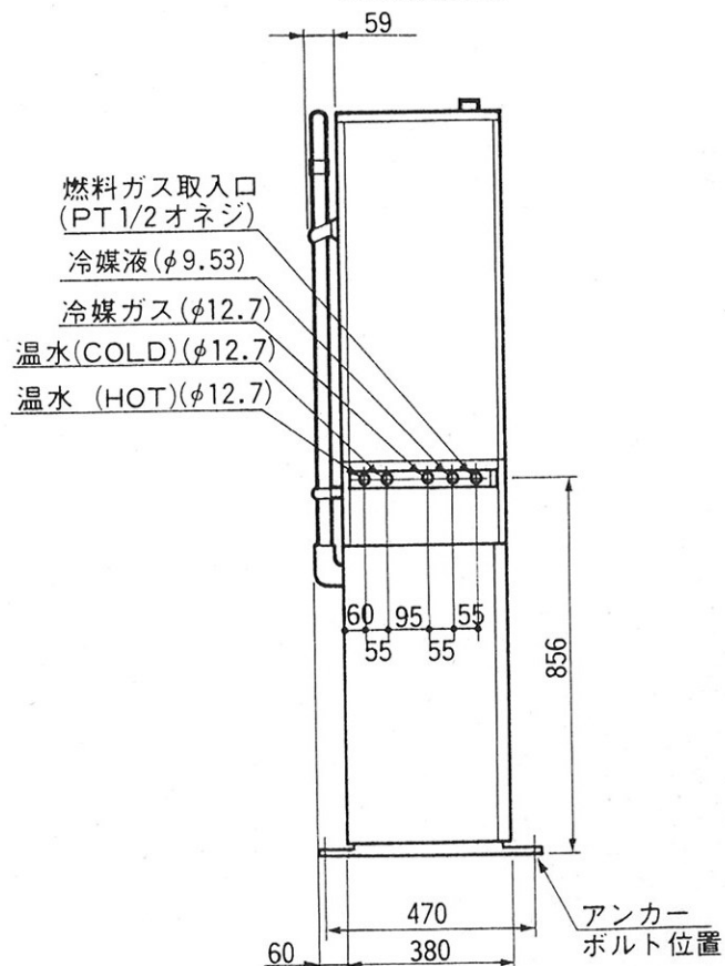
左側面図
