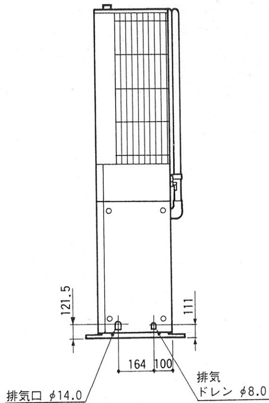
右側面図
