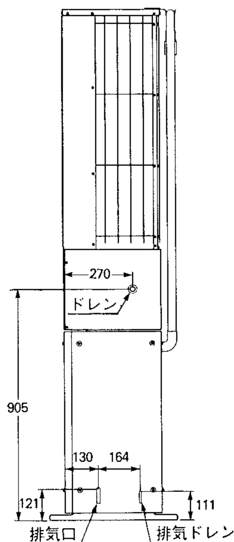
右側面図
