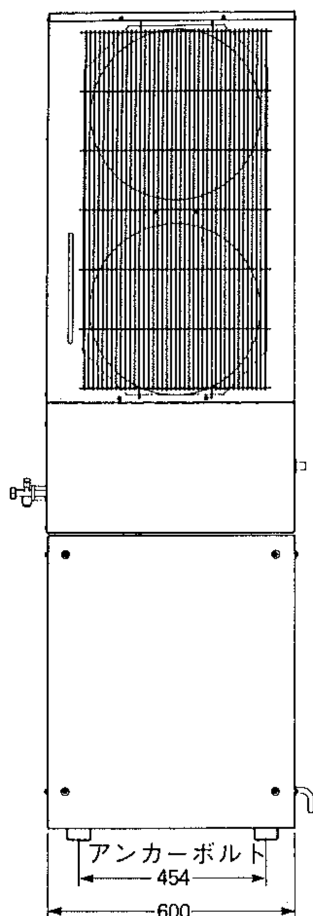
正面図
