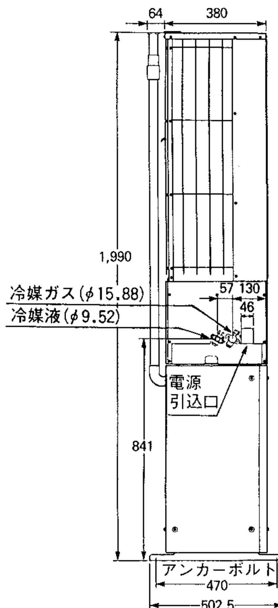
左側面図
