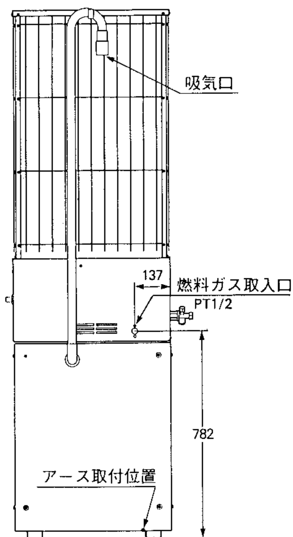
背面図
