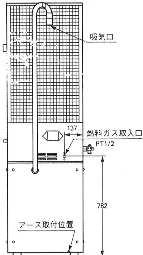
左側面図
