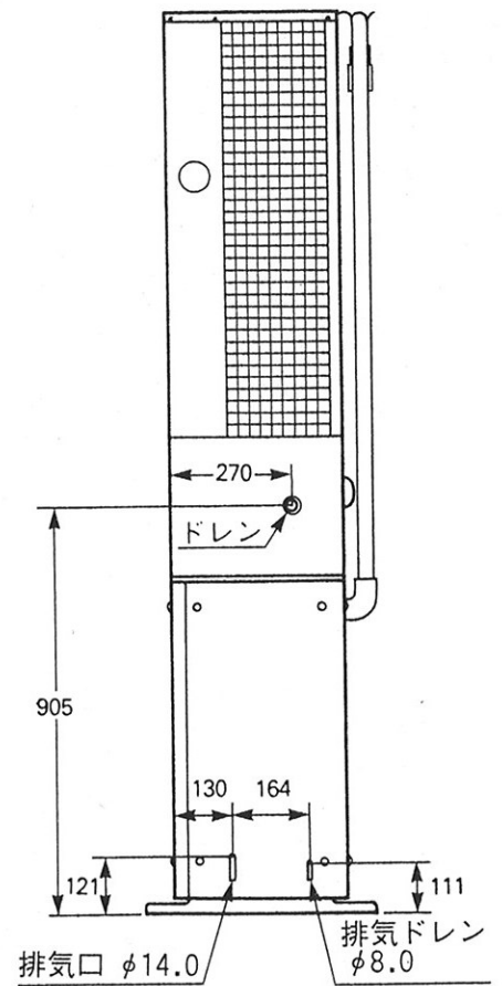
右側面図
