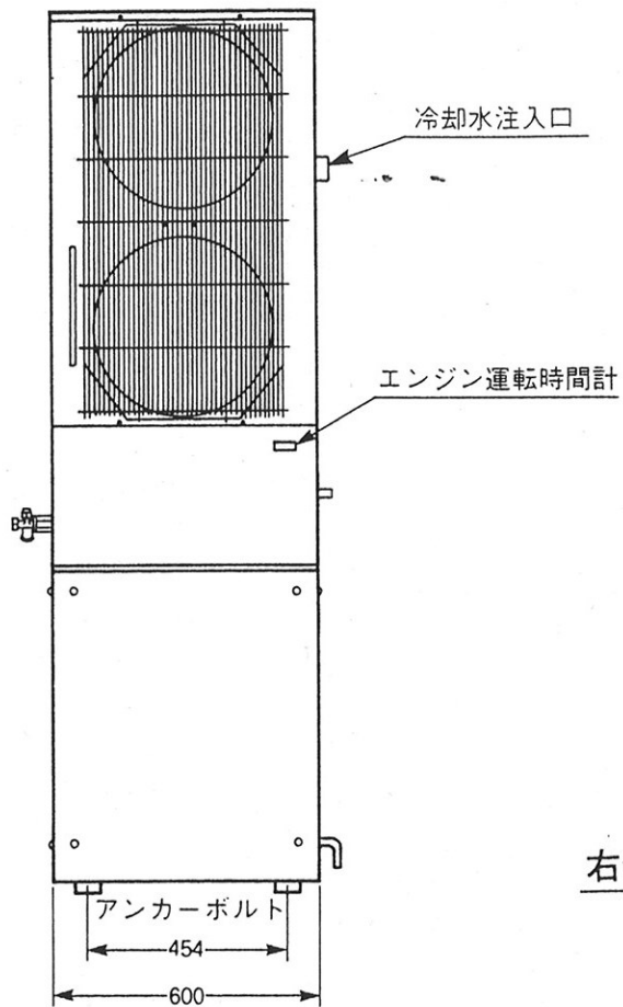
正面図
