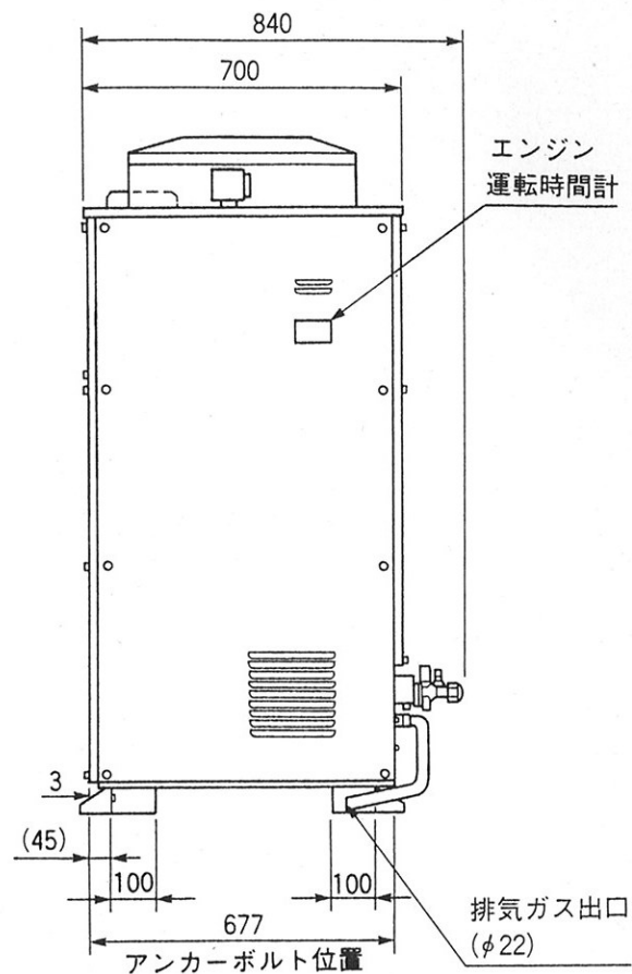
右側面図
