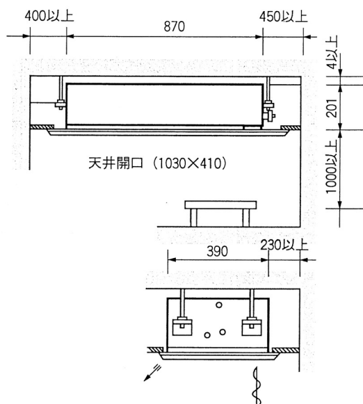
設置必要スペース
