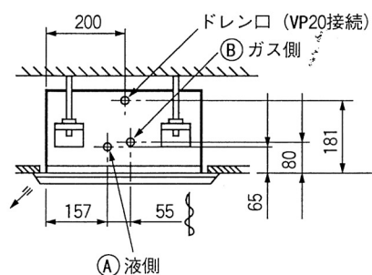
冷媒配管サイズ
