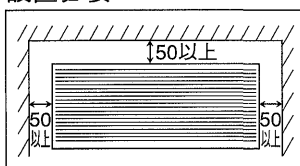
設置必要スペース
