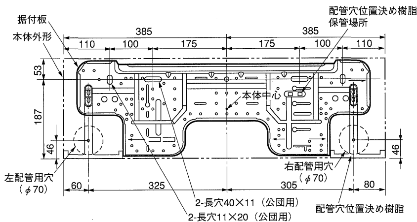
据付板位置関係〈正面図〉
