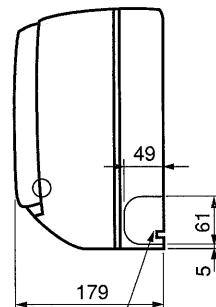
右配管用穴
