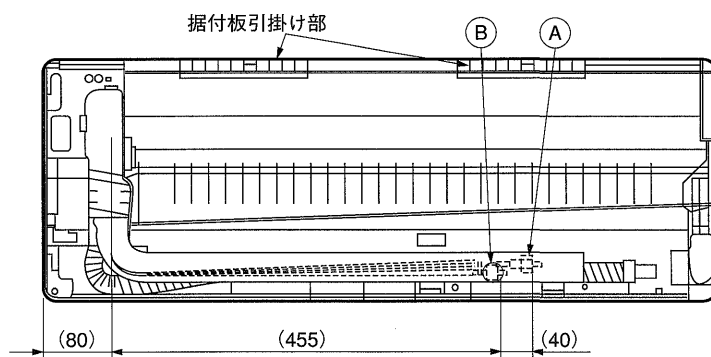
背面図
