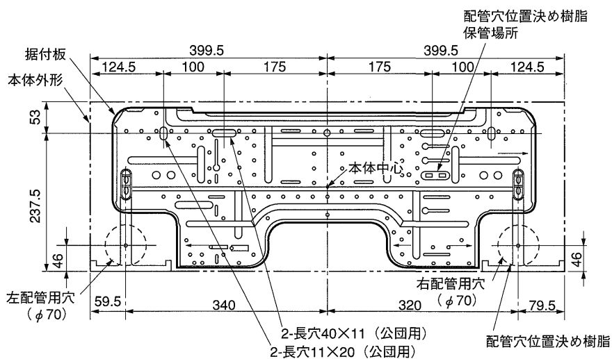
据付板位置関係〈正面図〉
