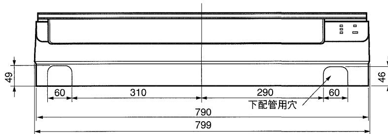
底面図
