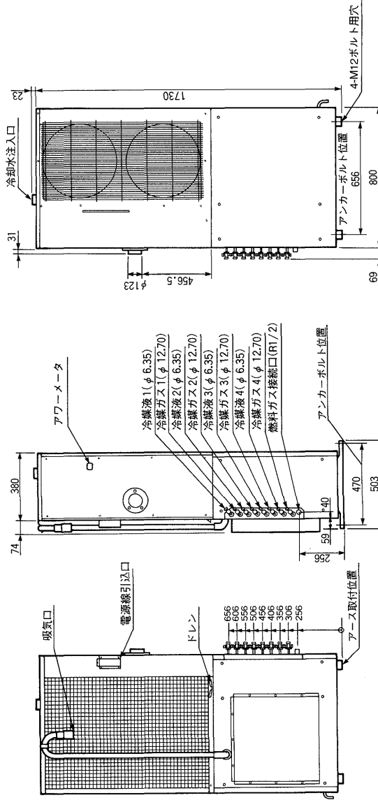
左側面図
