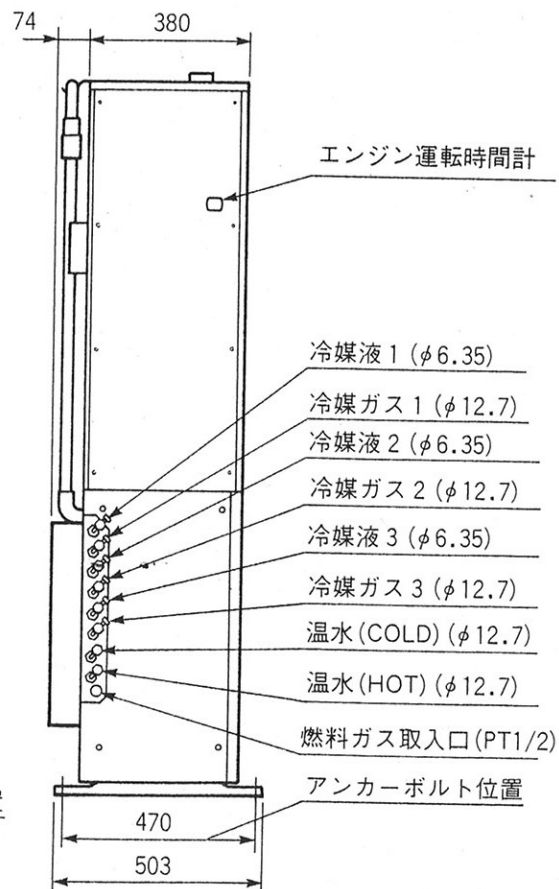
左側面図
