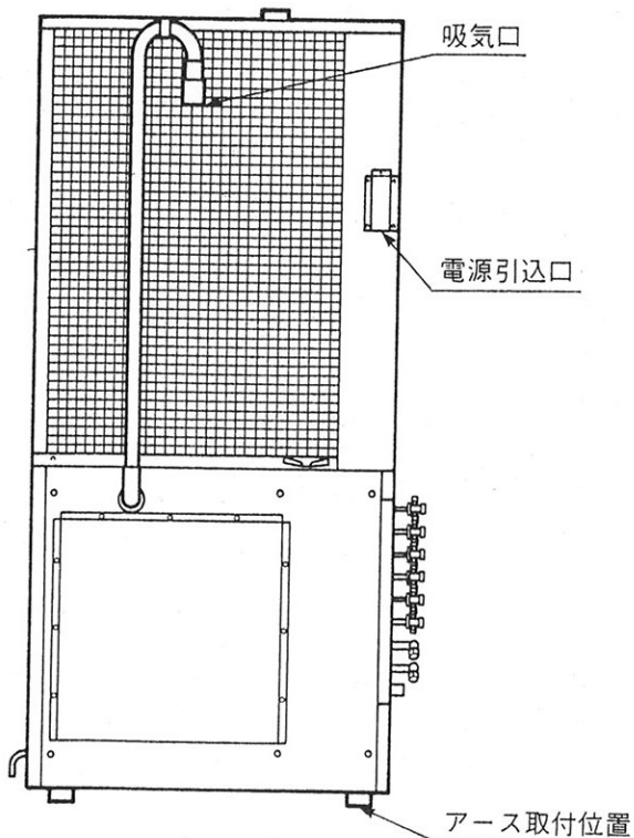
背面図
