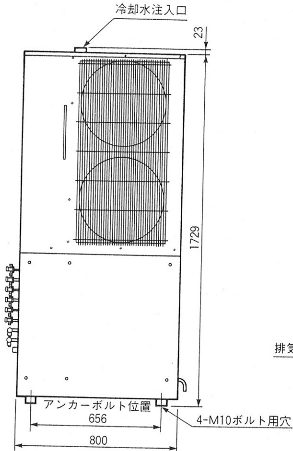
正面図
