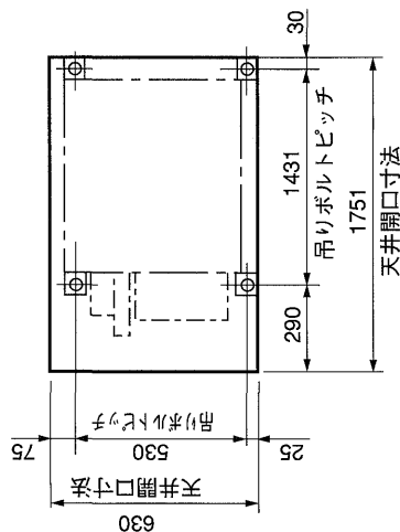
天井開口寸法 (Zから見る)
