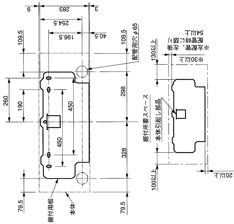
配管取り入れボルトタッピングネジ取付詳細
