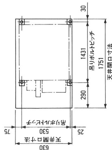
天井開口寸法 (Zカラ見ル)
