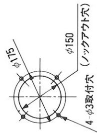
外気取入口詳細
