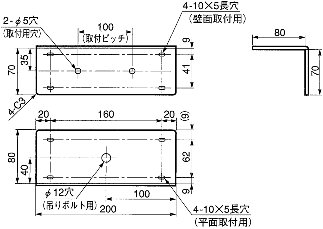
取付用金具
