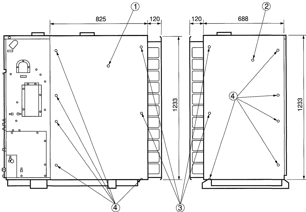
背面
