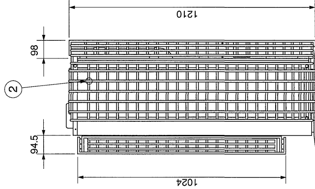
右側面
