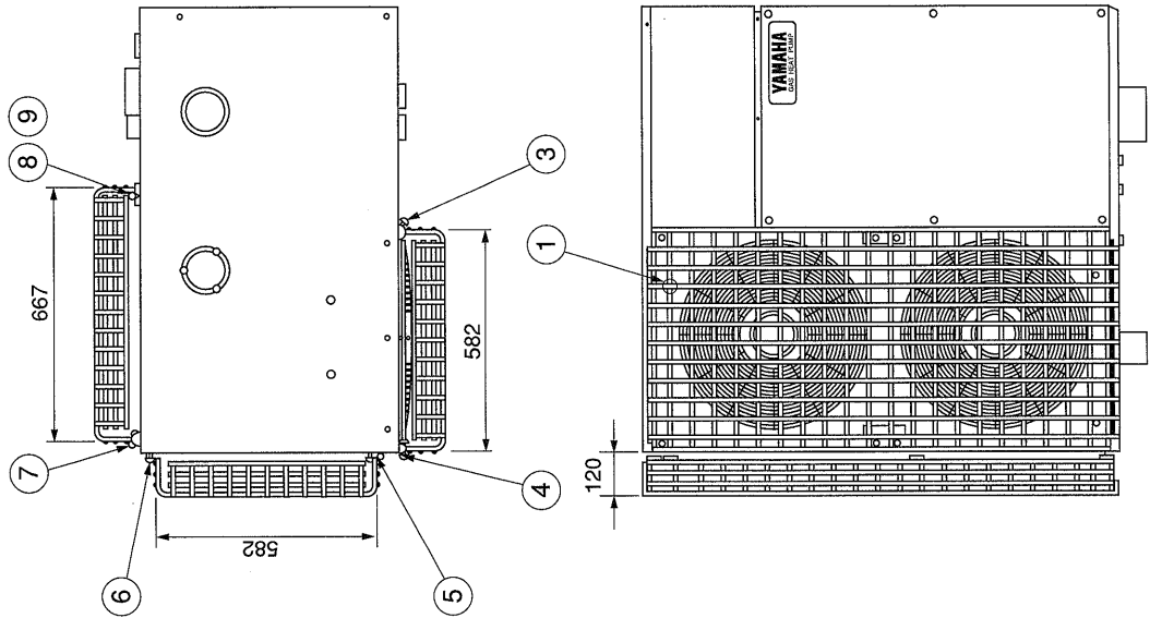
正面
