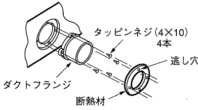
ダクトフランジ取付図
