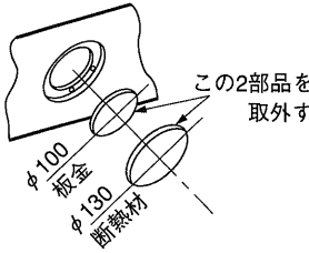
ノックアウト穴加工
