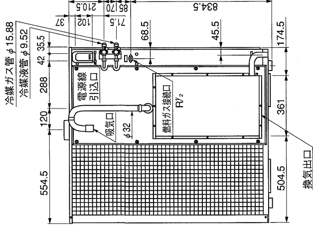
背面図
