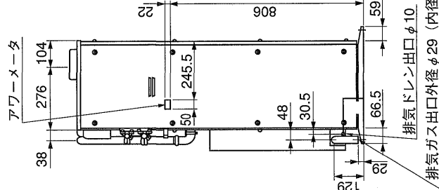
左側面図
