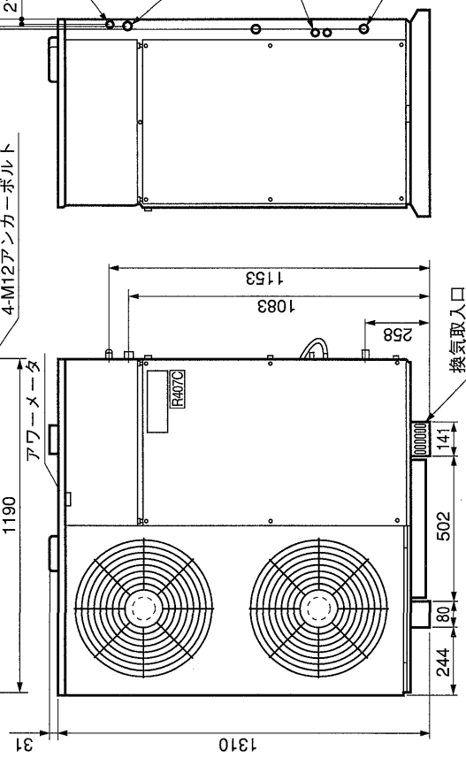
右側面図
