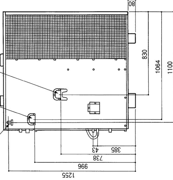
背面図
