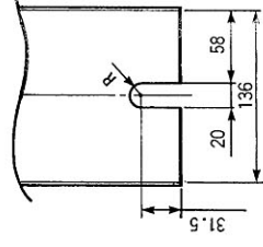
脚部詳細図
