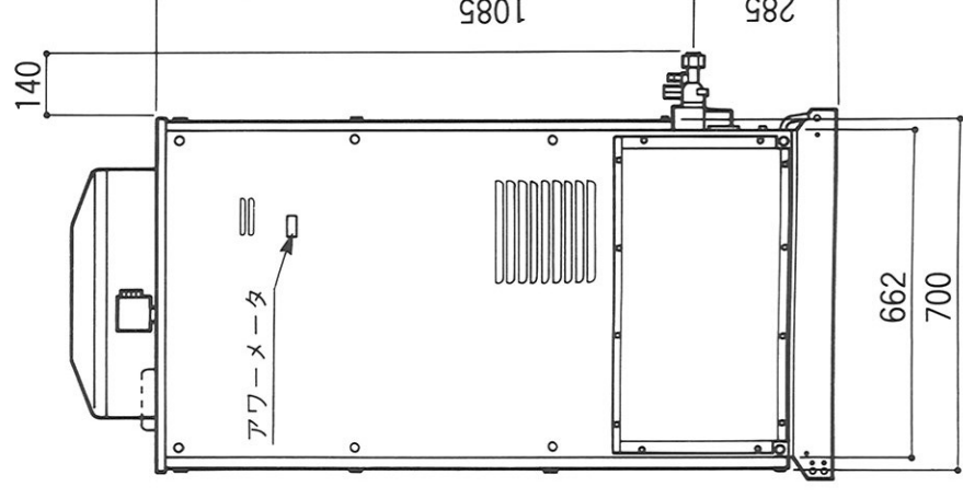
右側面図
