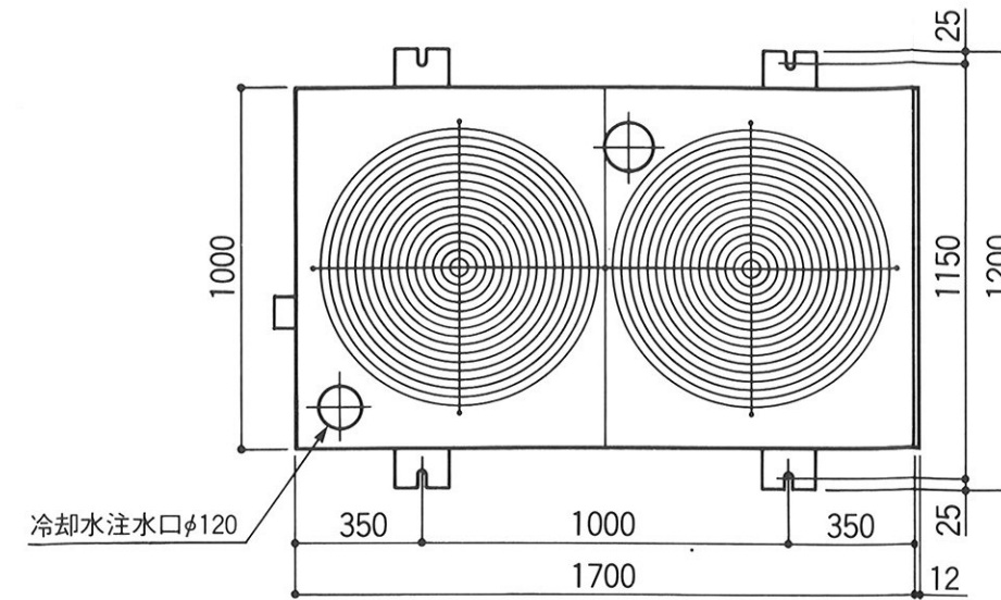
上面図
