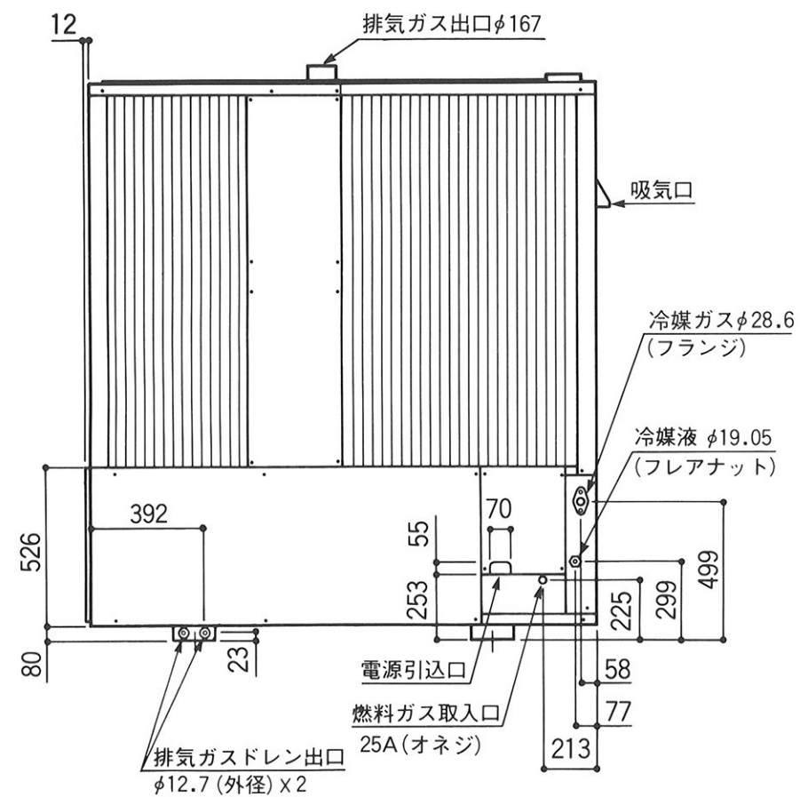
背面図
