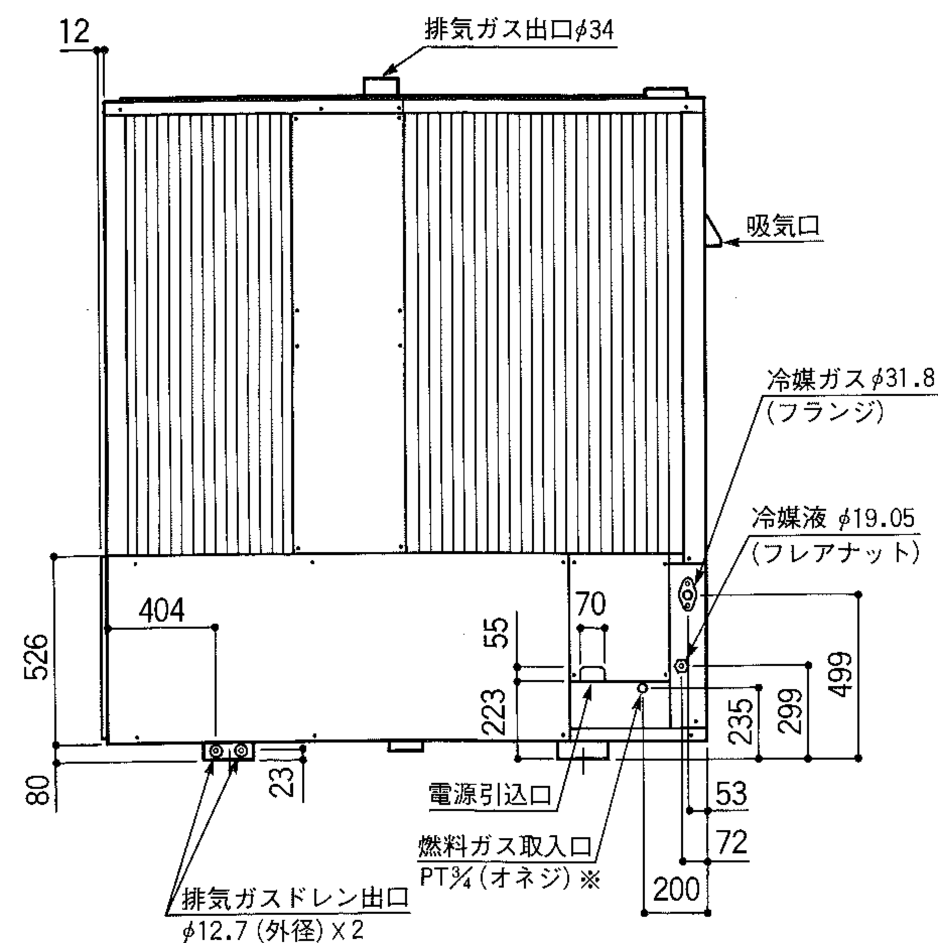
背面図
