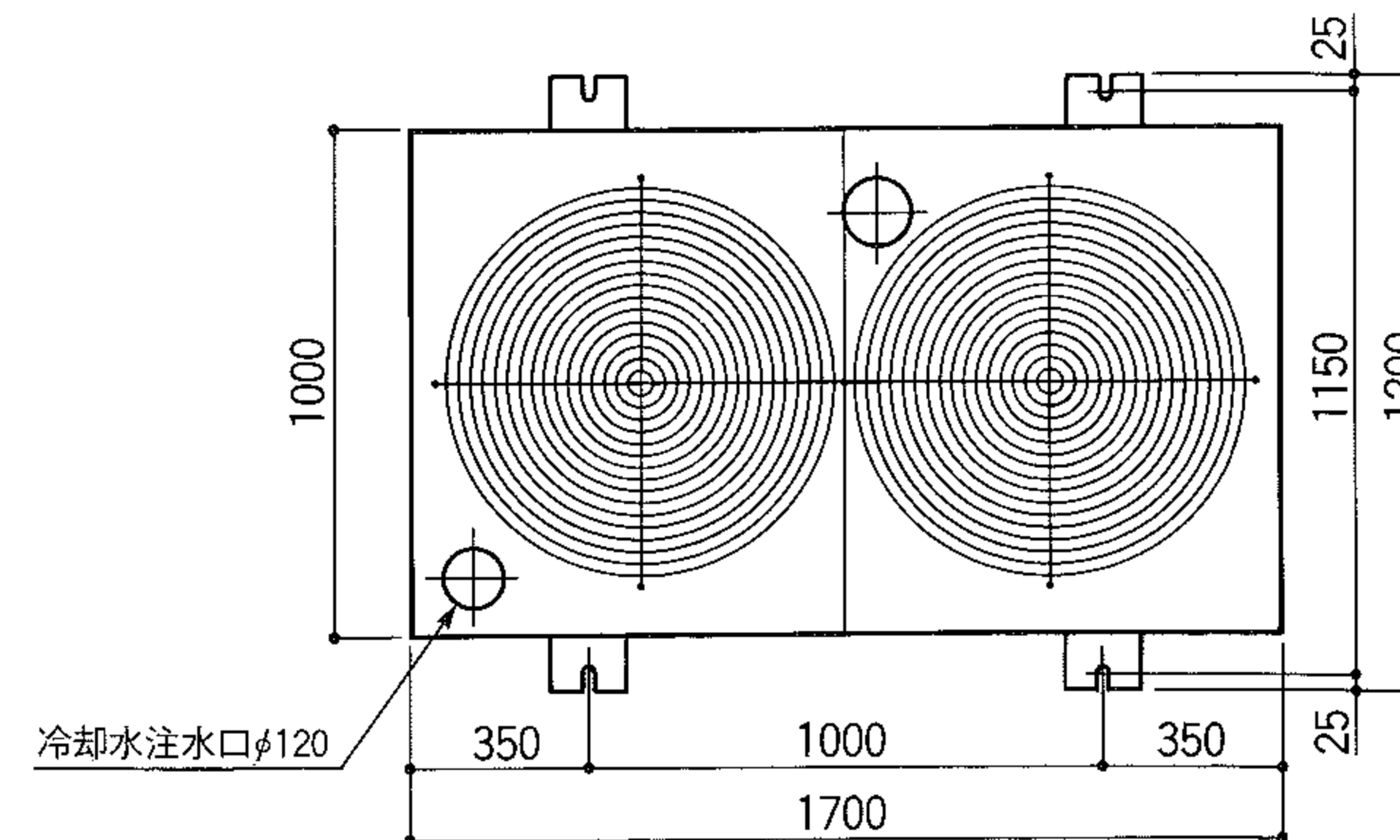
上面図
