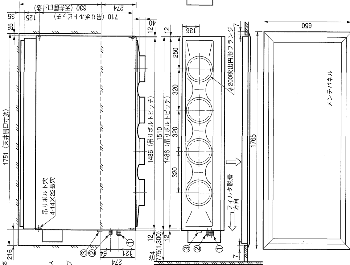
後吸込用フィルタボックス外形図
