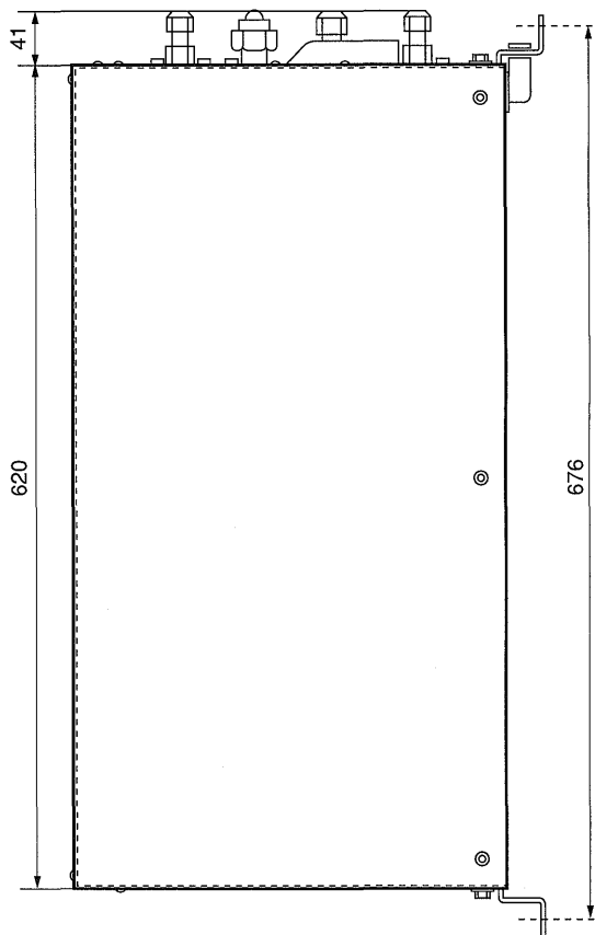
〈正面〉
