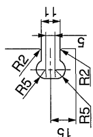
A部詳細
