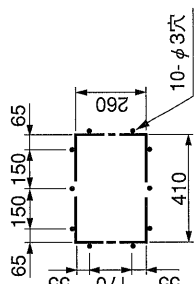
分ダクト穴詳細
