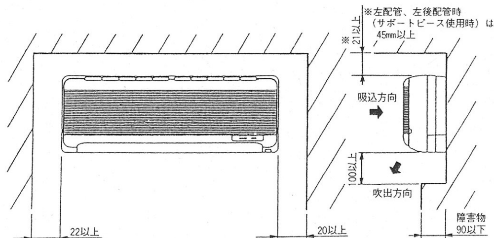
室内ユニット周囲必要空間
