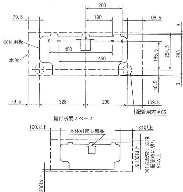
配管取り入れボルトタッピンネジ取付詳細
