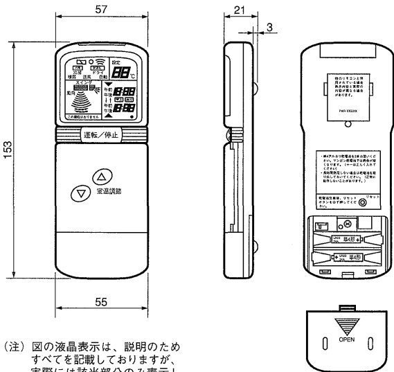
操作部
