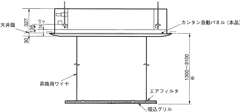
取付図(グリル下降時)
