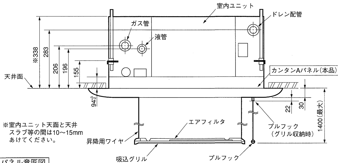
パネル意匠図
