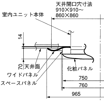
スペースパネルと併用の場合
