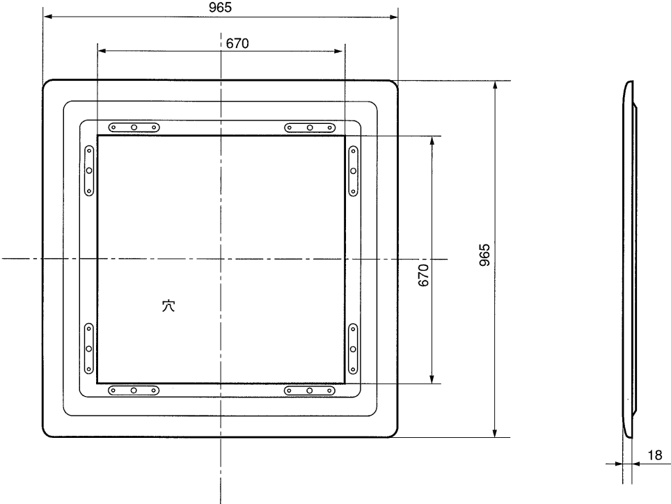
スペースパネルと併用の場合
