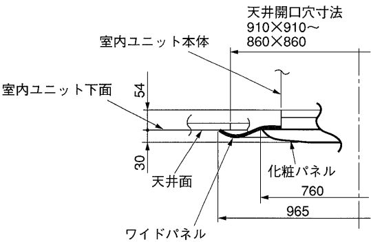
標準化粧パネルの場合
