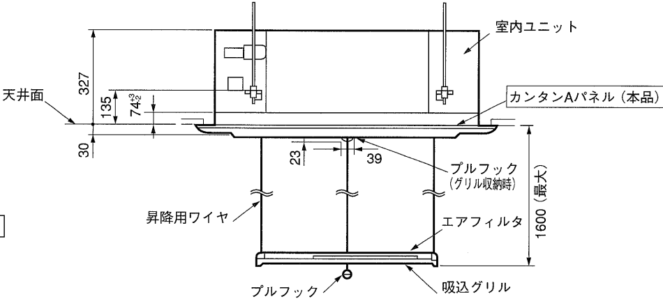
取付図(グリル下降時)
